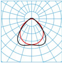
7850 HE PW40-120 ML 830 L150 12 50 ■ C0 - C180 DIN 5040 = A40 CEN flux code = 56 85 95 93 100 15 39 67 7 UGR I 3 = 23,7 UGR q 3 = 22,4 UTE 3 = 0.93 D + 0.07 T
