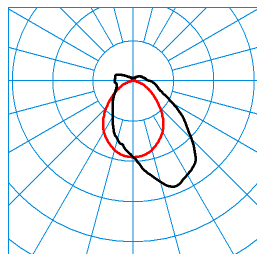
TugraHE 18 PAW 68-110/16ML-840 ET PC 23 (STAG13) TX425265 C0 - C180 C90 - C270 DIN 5040: B40 UTE: 0,86 E + 0,14 T CEN Flux Code: 48 77 92 86 100 13 32 64 14
