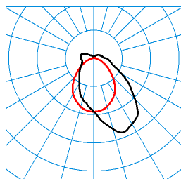
TugraHE 18 PAW 68-110/16ML-840 ET PC 23 (STAG11) TX425239 C0 - C180 C90 - C270 DIN 5040: B40 UTE: 0,86 E + 0,14 T CEN Flux Code: 48 77 92 86 100 13 32 64 14
