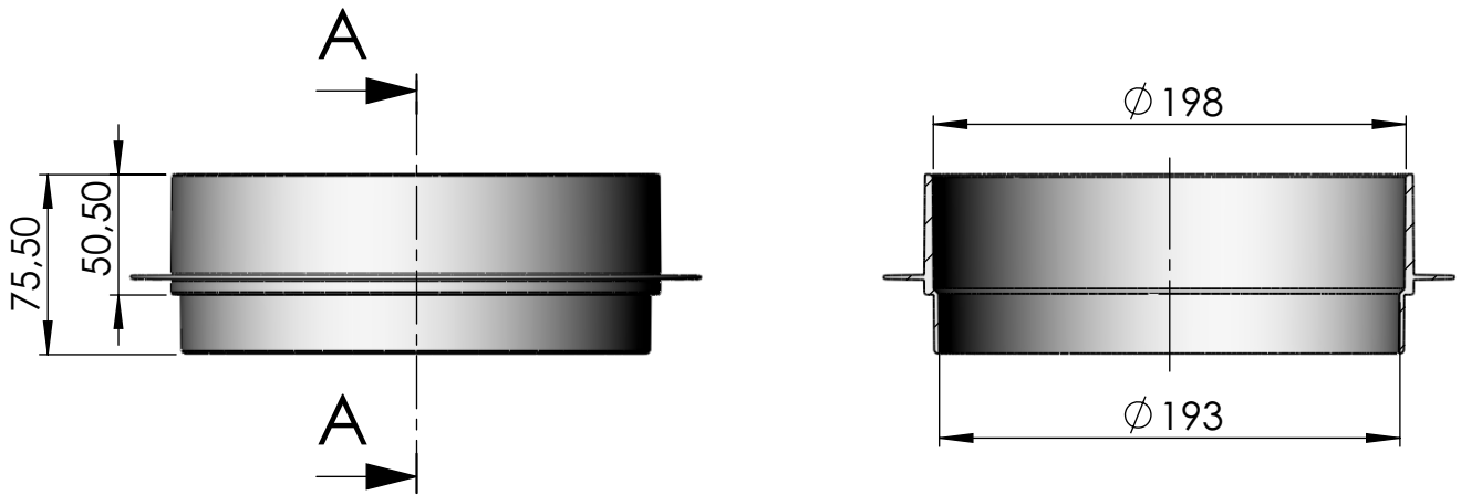
SECCIÓN A-A
