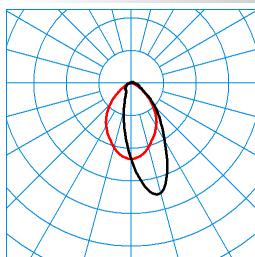
TX050655 DIN 5040: A50 UTE: 0,96 C + 0,04 T ■ C0 - C180 ■ C90 - C270
