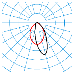
TX053193 DIN 5040: A50 UTE: 0,96 C + 0,04 T ■ C0 - C180 ■ C90 - C270
