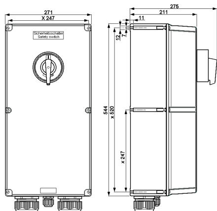
GHG 265..., 125 A 3- / 4- pôle GHG 266 ..., 180 A 3 pôle
