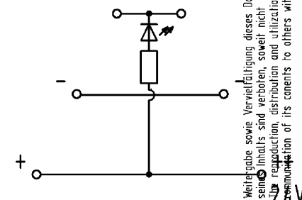
Schaltbild/diagram 57.503.9055.0
