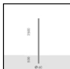
S.2800 POTEAU CYLINDRIQUE H 2,5m Ø60 mm À ENTERER Poteau cylindrique comprenant: fût droit à section circulaire, diamètre 60mm, épaisseur 3mm, longueur totale 3,00m, tronç unique construit en utilisant des tubes soudés à induction de façon longitudinale (ERW) UNI EN 10219-2-ISO 4200.
