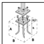
S.2849 Embase de fixation à sceller pour POTEAU S.2801, S.2813, S.2843, S.2845 à sceller en acier zingué avec visserie M16, C= 200mm, D=200mm E=Ø80mm, h=460mm, h1=90mm. Il est conseillé de sceller cette embase dans le béton selon les dimensions ci-dessous **: A = 0.7 m B = 0.7 m **Les dimensions du bloc de béton peuvent varier en fonction de la nature du terrain, selon les indications de la norme UNI EN 40.
