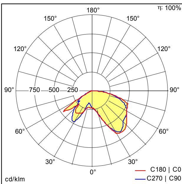
D43627_RESC_PRO_TEC-GP_ESC90_ECD_WH.Idt
