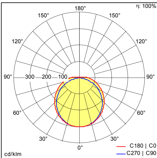
TLX_S_3000-840_O_END_L.idt
