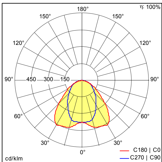
D41246AA_TECTON_C_LED3700-830_L1000_VWB_LDE_BK.ltd
