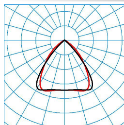
ELINE LN140 865 L225 1 20
