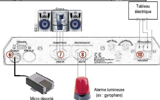
Schéma de câblage pour alimentation directe d'une sono ( P_{max} \leq 2000\text{ W} )
