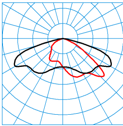
Jovie 70-AB7L-LR/16500-730 18G1 ET TX068606 ■ C0 - C180 ■ C90 - C270 DIN 5040: A30 UTE: 1,00 G CEN Flux Code: 35 72 97 100 100
