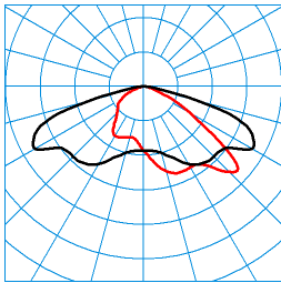
Jovie 70-AB7L-LR/16500-730 18G1 ET (CLO end value) TX300636 ■ C0 - C180 ■ C90 - C270 DIN 5040: A30 UTE: 1,00 G CEN Flux Code: 35 72 97 100 100
