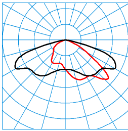
Jovie 70-AB7L-LR/16500-730 18G1 ET (CLO initial value) TX301283 ■ C0 - C180 ■ C90 - C270 DIN 5040: A30 UTE: 1,00 G CEN Flux Code: 35 72 97 100 100
