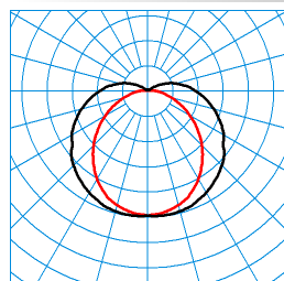
Kratex NS HE 0.6 20-840 ET PC TX199200
