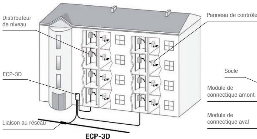
ECP-3D Alimentation de deux colonnes
