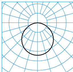
Skeo Circ MultiLC WD1 1G1Y ET (cw) ■ C0 - C180 TX278625 UGR I = 22,9 UGR q = 22,9 DIN 5040: A40 UTE: 1,00 E CEN Flux Code: 47 78 96 100 100
