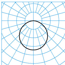
Skeo Circ MultiLC WD1 1G1Y ET (nw) ■ C0 - C180 TX278619 UGR I = 24,2 UGR q = 24,2 DIN 5040: A40 UTE: 1,00 E CEN Flux Code: 47 78 96 100 100
