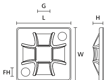
Embase Série QM
