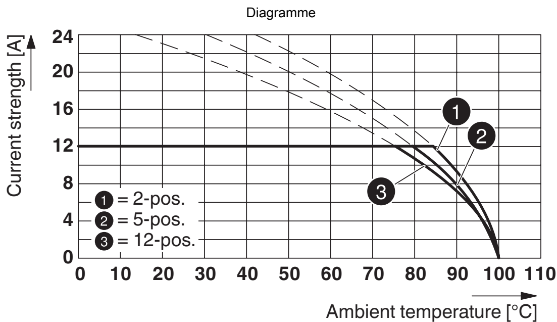
Type : FKC 2,5/...-ST-5,08 avec CCV 2,5/...-G-5,08 P26THR
