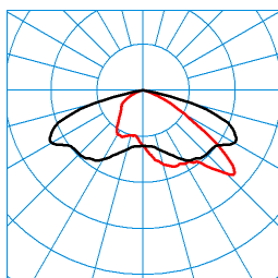
LnPlus 60-AB7L-LR/26000-722 24G1 ET (CLO initial value) TX390182 ■ C0 - C180 ■ C90 - C270 DIN 5040: A30 UTE: 1,00 G CEN Flux Code: 35 73 98 100 100
