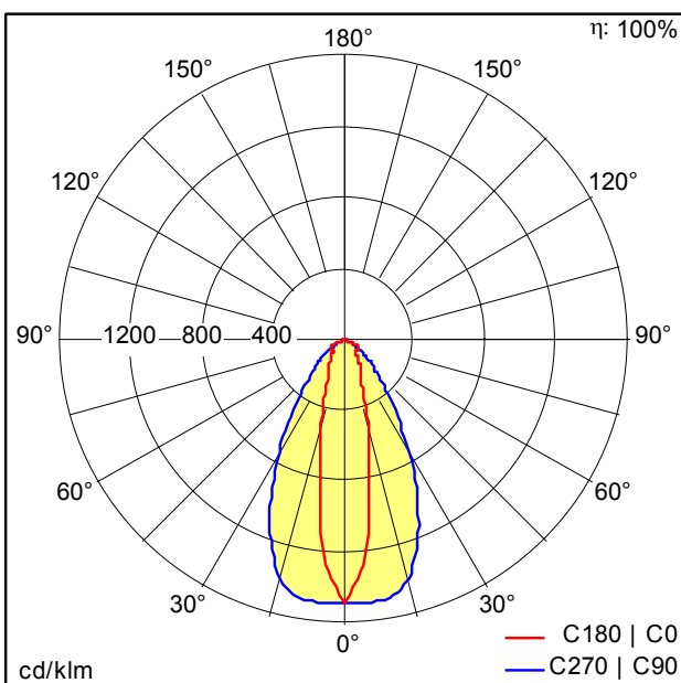
D44423AA_TEC_LED7400-865_L2000_NB_LDE_SR_IP.ltd
