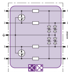
Schéma de principe du circuit BXT ML4 BE 36
