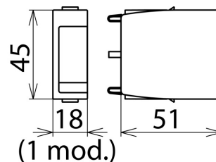
Dimensions DG MOD 440
