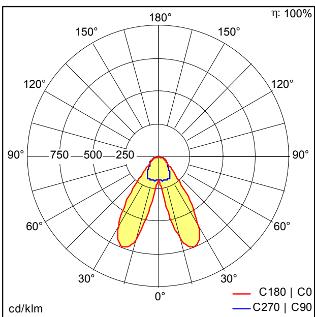
D43655AA_TECTON_C_LED3700-830_L1000_SB_LDE_WH.Idt
