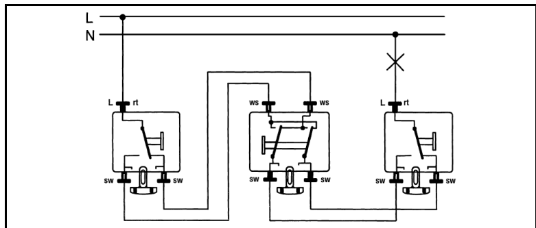
Schémas de raccordement
