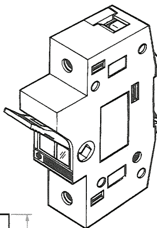
GK1-E●
