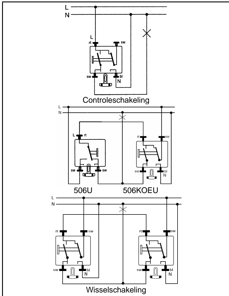
Schakelschema 506 KOEU
