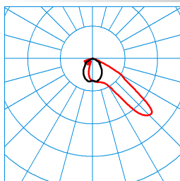
Jovie 50I-AM2L-LRA/4200-730 4G1 ET TX195507 ■ C0 - C180 ■ C90 - C270 DIN 5040: A40 UTE: 1,00 F CEN Flux Code: 47 91 100 100 100
