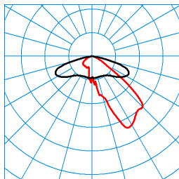
Publisca P1-AB2L-LR/2900-740 4G1S ET (CLO end value) TX300379
