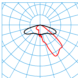
Publisca P1-AB2L-LR/2900-740 4G1S ET (CLO initial value) TX300538
