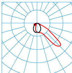
Jovie 50I-AM2L-SLR3/6800-730 6G1 ET (CLO initial value) TX300195 ■ C0 - C180 ■ C90 - C270 DIN 5040: A40 UTE: 1,00 F CEN Flux Code: 47 91 100 100 100
