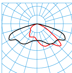
Jovie 70-AB7L-LRA/16500-740 18G1 ET (CLO initial value) TX301598 ■ C0 - C180 ■ C90 - C270 DIN 5040: A30 UTE: 1,00 G CEN Flux Code: 35 72 97 100 100
