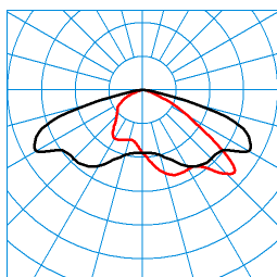
Jovie 70-AB7L-LRA/16500-740 18G1 ET (CLO end value) TX301231 ■ C0 - C180 ■ C90 - C270 DIN 5040: A30 UTE: 1,00 G CEN Flux Code: 35 72 97 100 100
