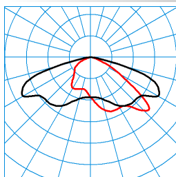
Jovie 70-AB7L-LRA/16500-740 18G1 ET TX068631 ■ C0 - C180 ■ C90 - C270 DIN 5040: A30 UTE: 1,00 G CEN Flux Code: 35 72 97 100 100
