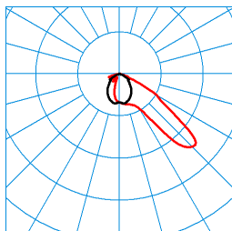
Jovie 50I-AM2L-SLR2/6800-730 6G1 ET (CLO initial value) TX300592 ■ C0 - C180 ■ C90 - C270 DIN 5040: A40 UTE: 1,00 F CEN Flux Code: 47 91 100 100 100
