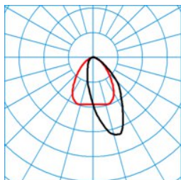
7850 HE LAN60-160 ML 830 L225 10 50 ■ C0 - C180
