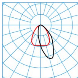
7850 HE LAN60-160 ML 830 L225 12 50 ■ C0 - C180
