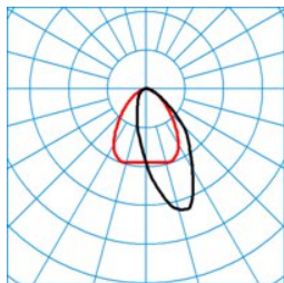
7850 HE LAN60-160 ML 830 L225 14 50 ■ C0 - C180
