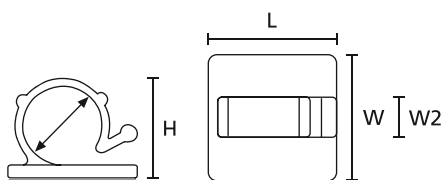
Série RA (vue de côté)
