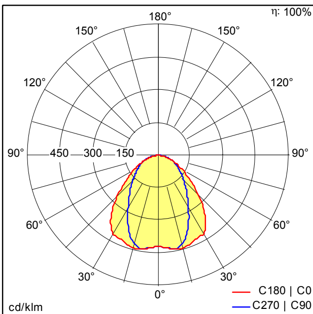
D44422AA_TEC_LED16000-840_L2000_VWB_LDE_WH_IP.idt
