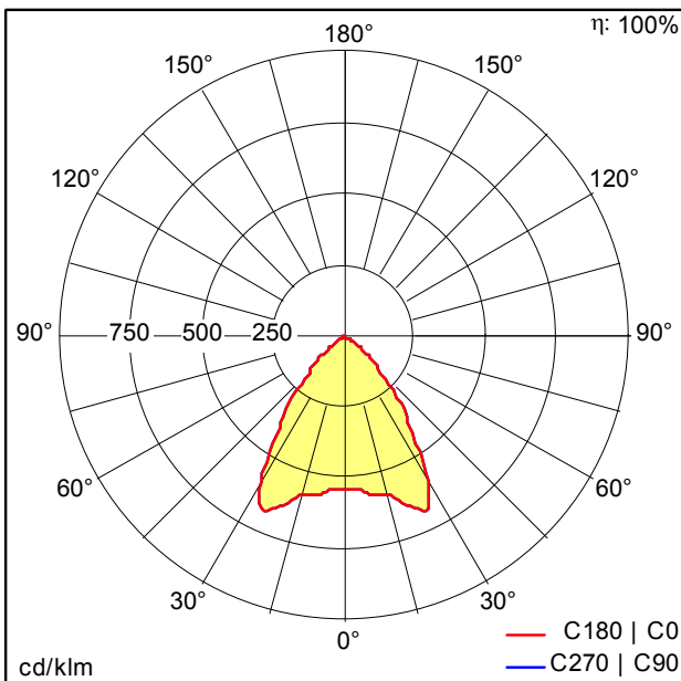
D35587AA_MIRL_MINI_EM_LED1200-840_EVG.ltd (mesure provisoire)
