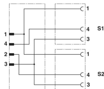
Schaltplan
