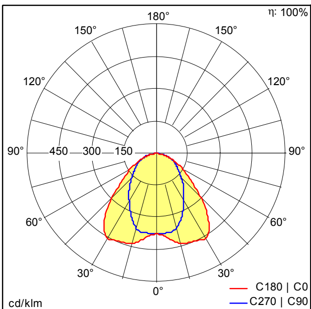
D41246AA_TECTON_C_LED7400-830_L2000_VWB_LDE_SR.Idt
