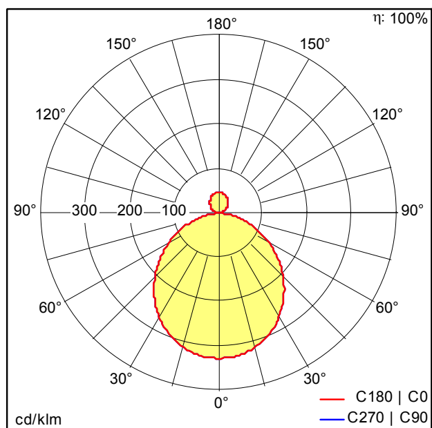
D38337AA_ONDA2_P_AV_D590_LED3000-830.idt
