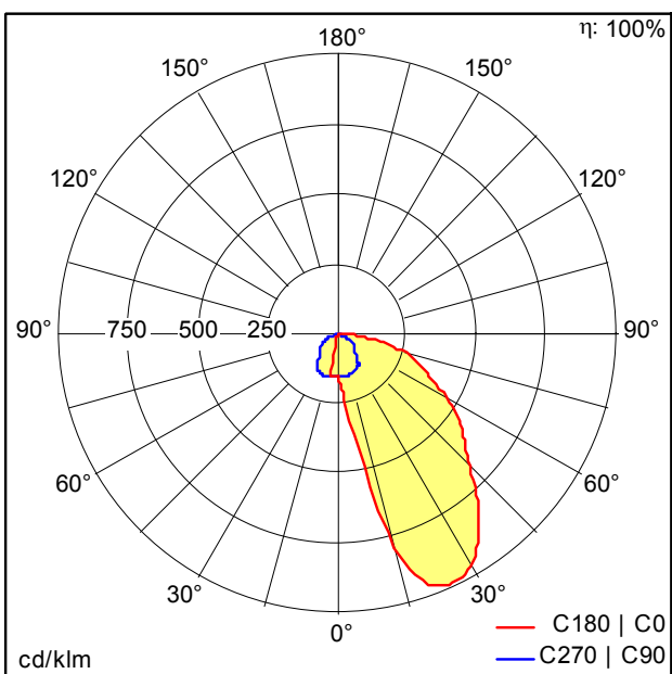
D34983AA_TECTON_C_LED10000-840_L2000_WW_EVG_WH.Idt
