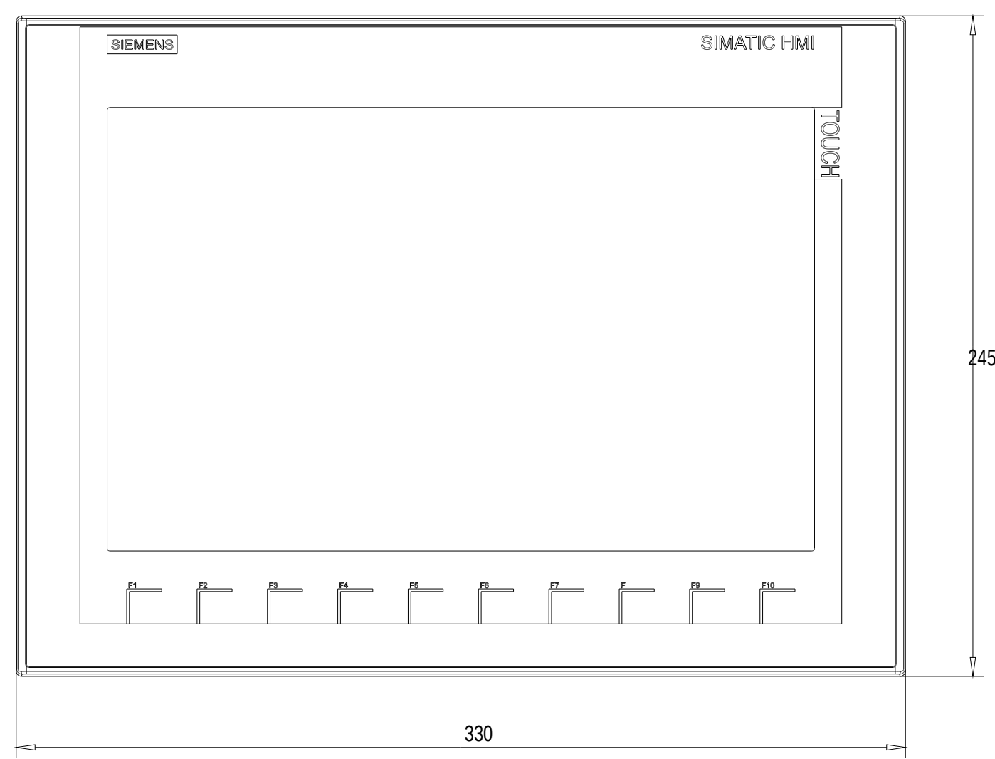
Vorne / Front
