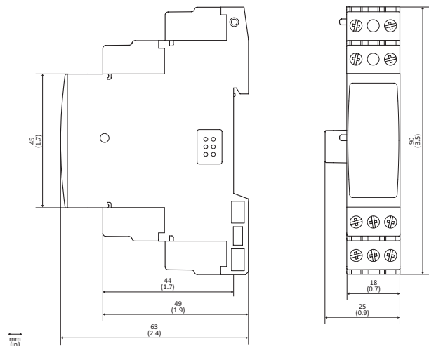
Fig. 2 Dimensions VMU-OC
