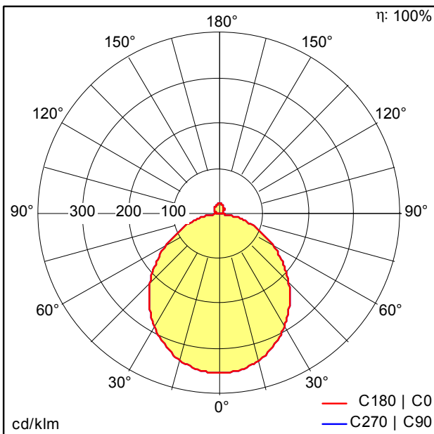
D38339AA_ONDA2_AV_D1150_LED7000-927-65_WH.Idt
