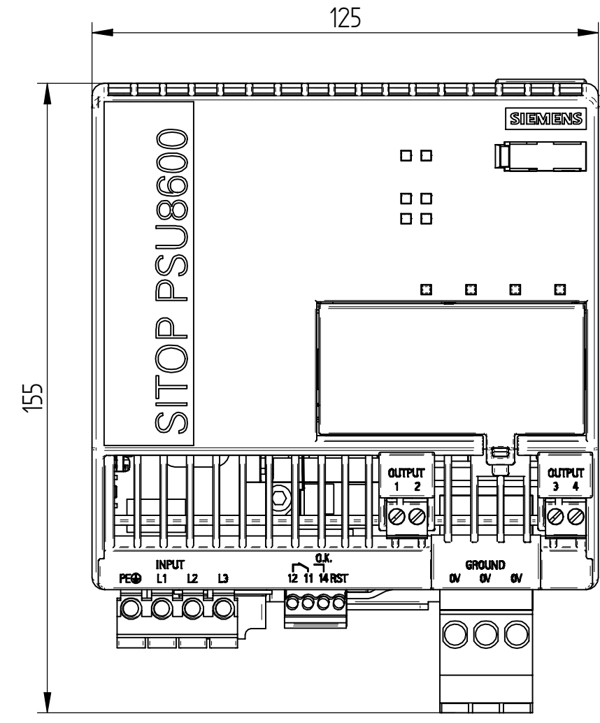
Vorne / Front
