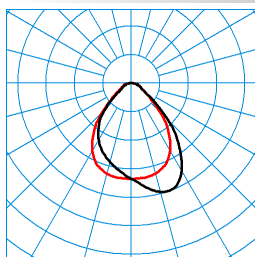
ArimoFit G2 Act D2 P-WW 42-8 ETDD8 01/01 (ACTDWW) TX377112 ■ C0 - C180 ■ C90 - C270 DIN 5040: A50 UTE: 1,00 C CEN Flux Code: 66 90 97 100 100
