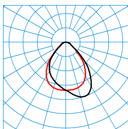
ArimoFit G2 Act D2 P-WW 42-8 ETDD8 01/01 (ACTDSU) TX377596 ■ C0 - C180 ■ C90 - C270 DIN 5040: A50 UTE: 1,00 C CEN Flux Code: 66 90 97 100 100
