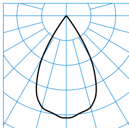
Kalo G2 3P RF-VFL-c 20-M+F M53 ETDD 01 TX823565
