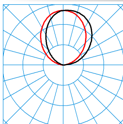
Sanesca W2 LED2600-840 03 TX371855 ■ C0 - C180 ■ C90 - C270 DIN 5040: E03 UTE: 0,00 J + 1,00 T CEN Flux Code: 0 0 0 0 100 51 81 96 100
