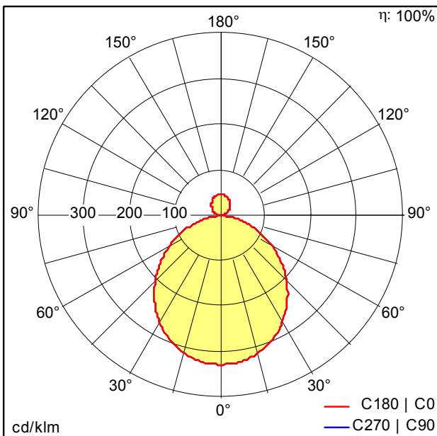
D38337AA_ONDA2_AV_D590_LED2000-927-65_WH.Idt
