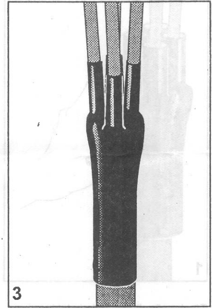
3 Bien chauffer entre les conducteurs. L'extrémité est terminée lorsque un filet d'adhésif déborde sur les isolants du câble et des conducteurs.
