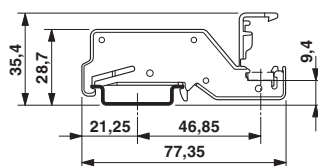
Dessin coté
