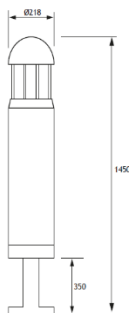
VERSION ANCRAGE RENFORCE (scellement béton)
